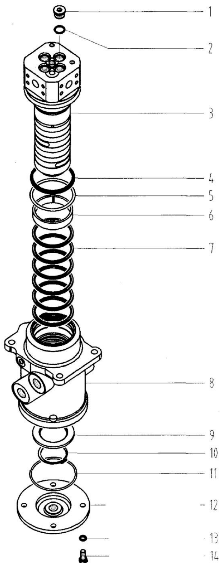
Центральное соединение
