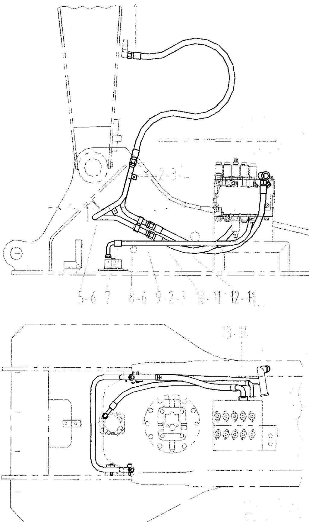
Основной трубопровод гидромолота на раме
