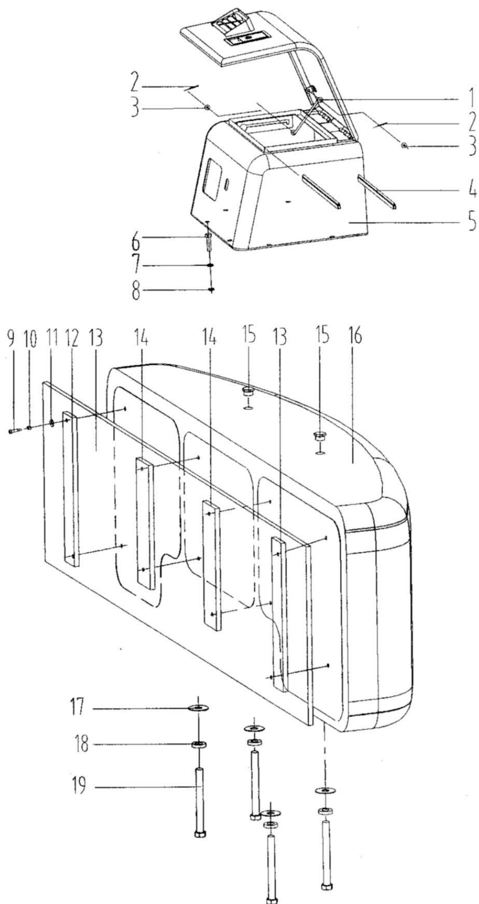
Ящик с инструментами и противовес
