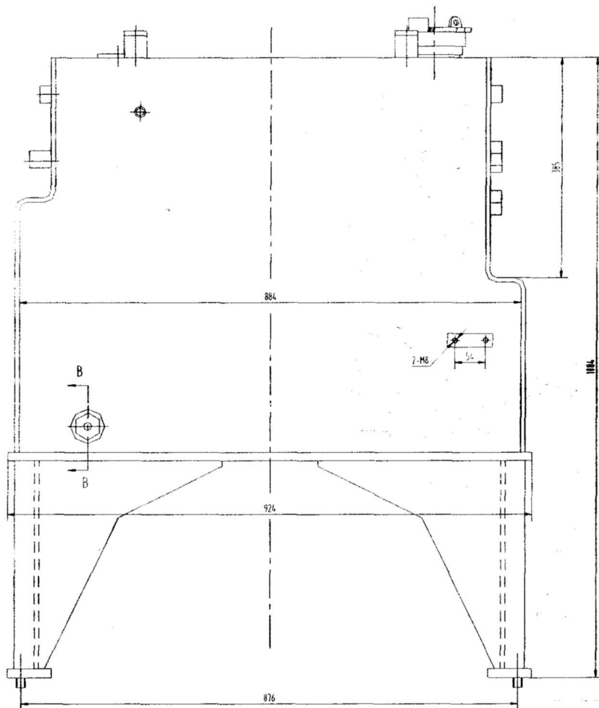
00E1075 Бак топливный в сборе
