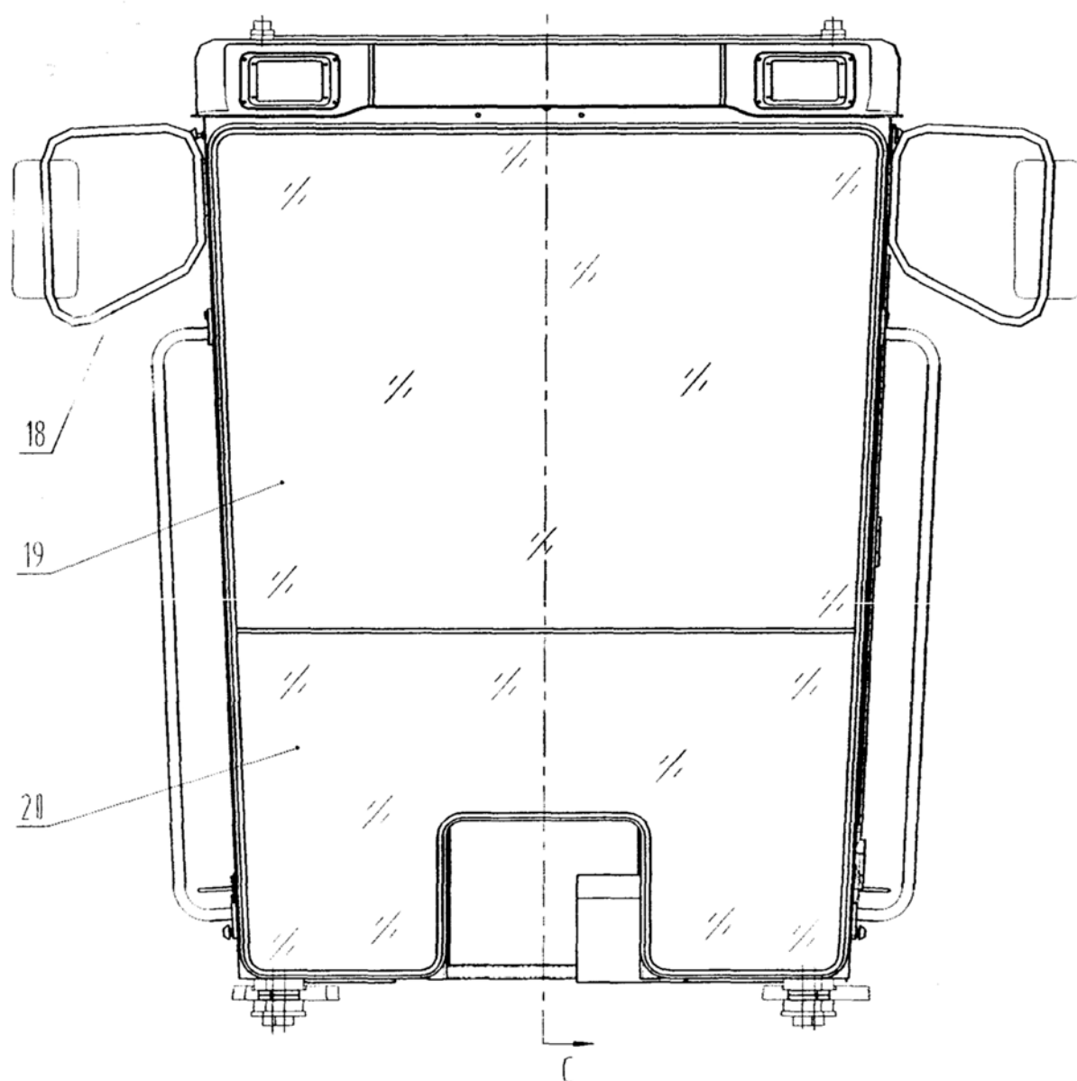
41E0062 Кабина в сборе
