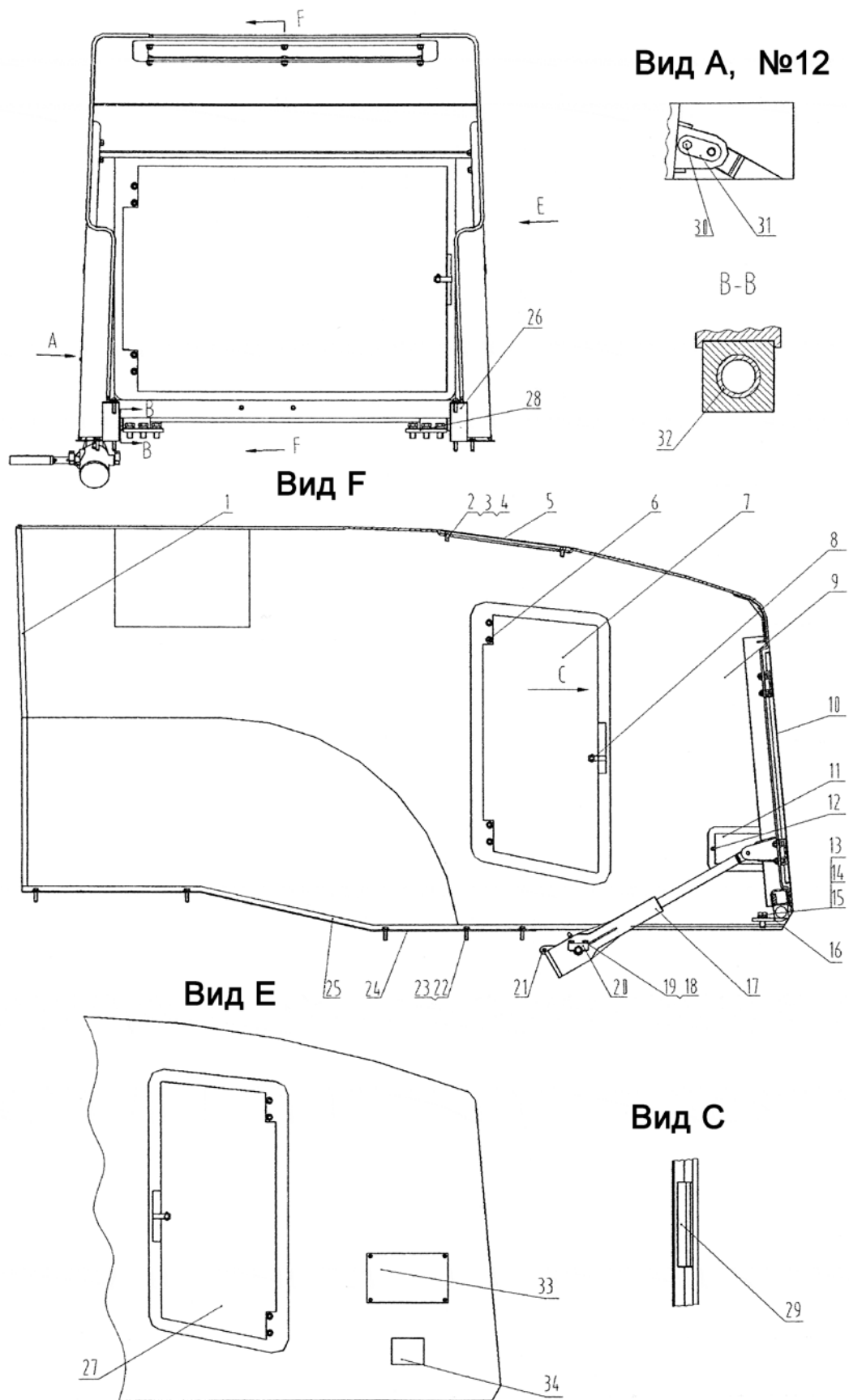
44E0027 Капот двигателя
