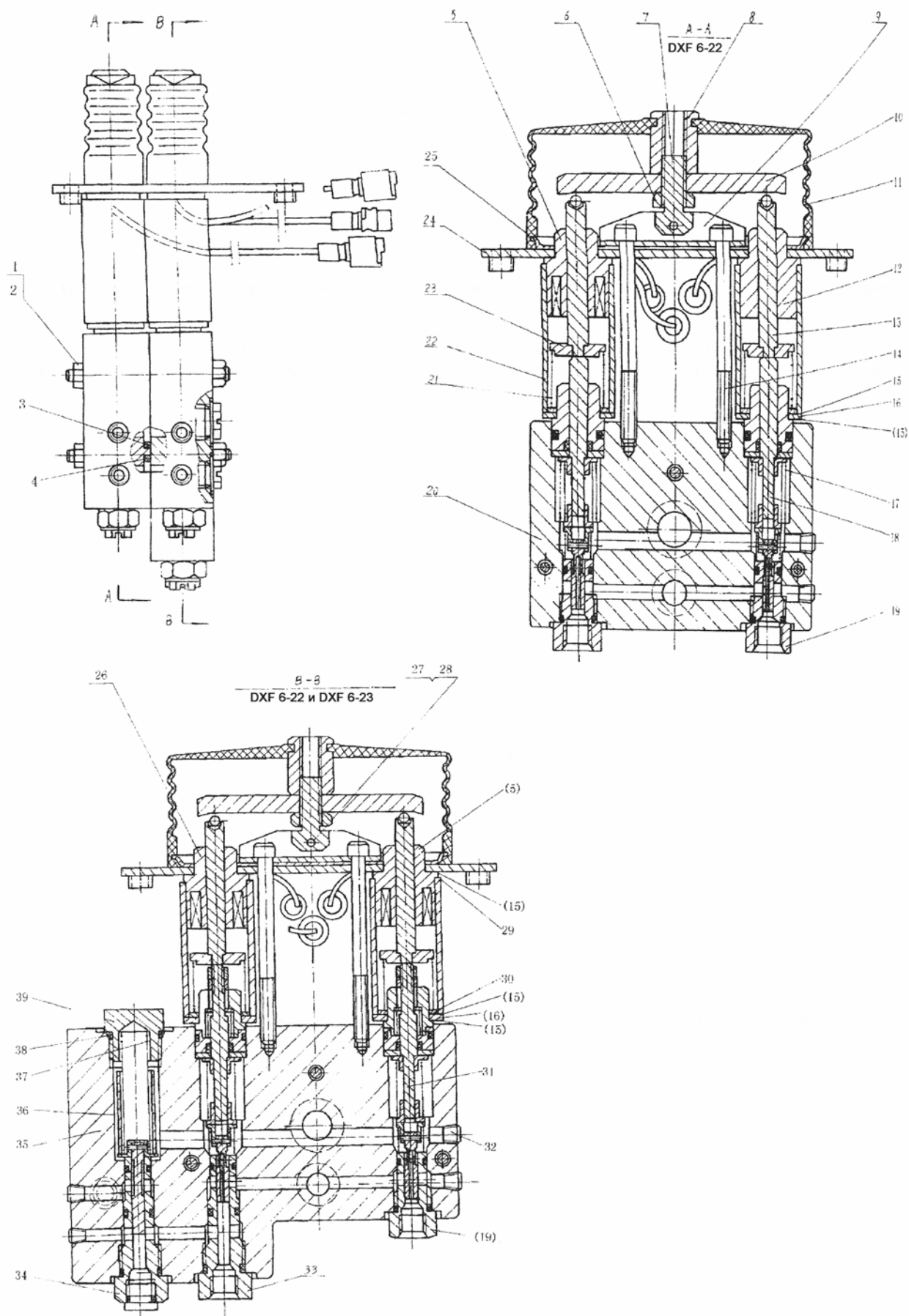
ХДФ6 Клапан управляющий
