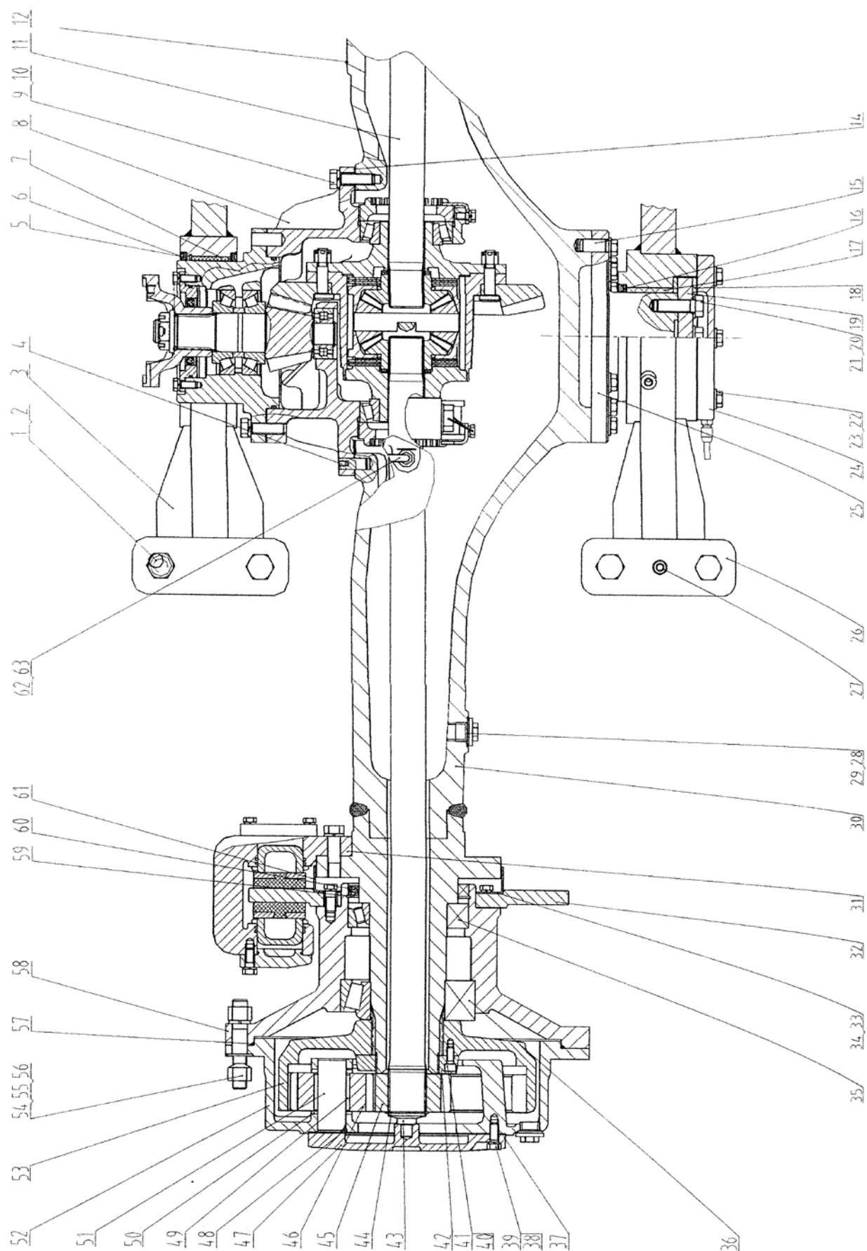
01E0022 Мост задний в сборе
