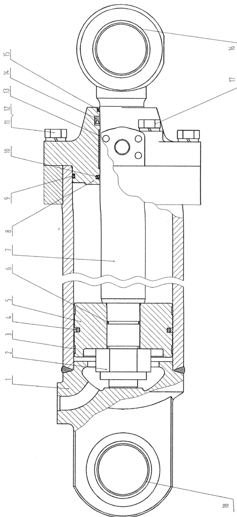
10C0024 Гидроцилиндр опрокидывания
