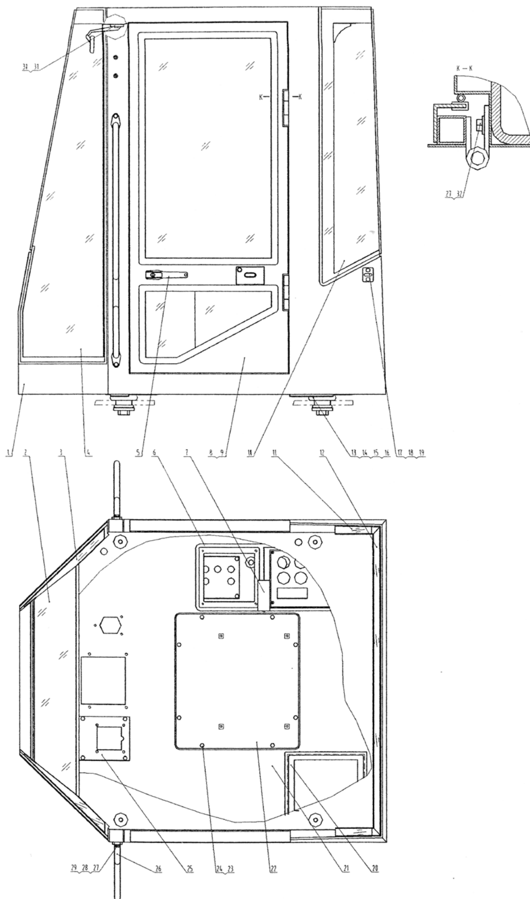
41E0006 Кабина в сборе
