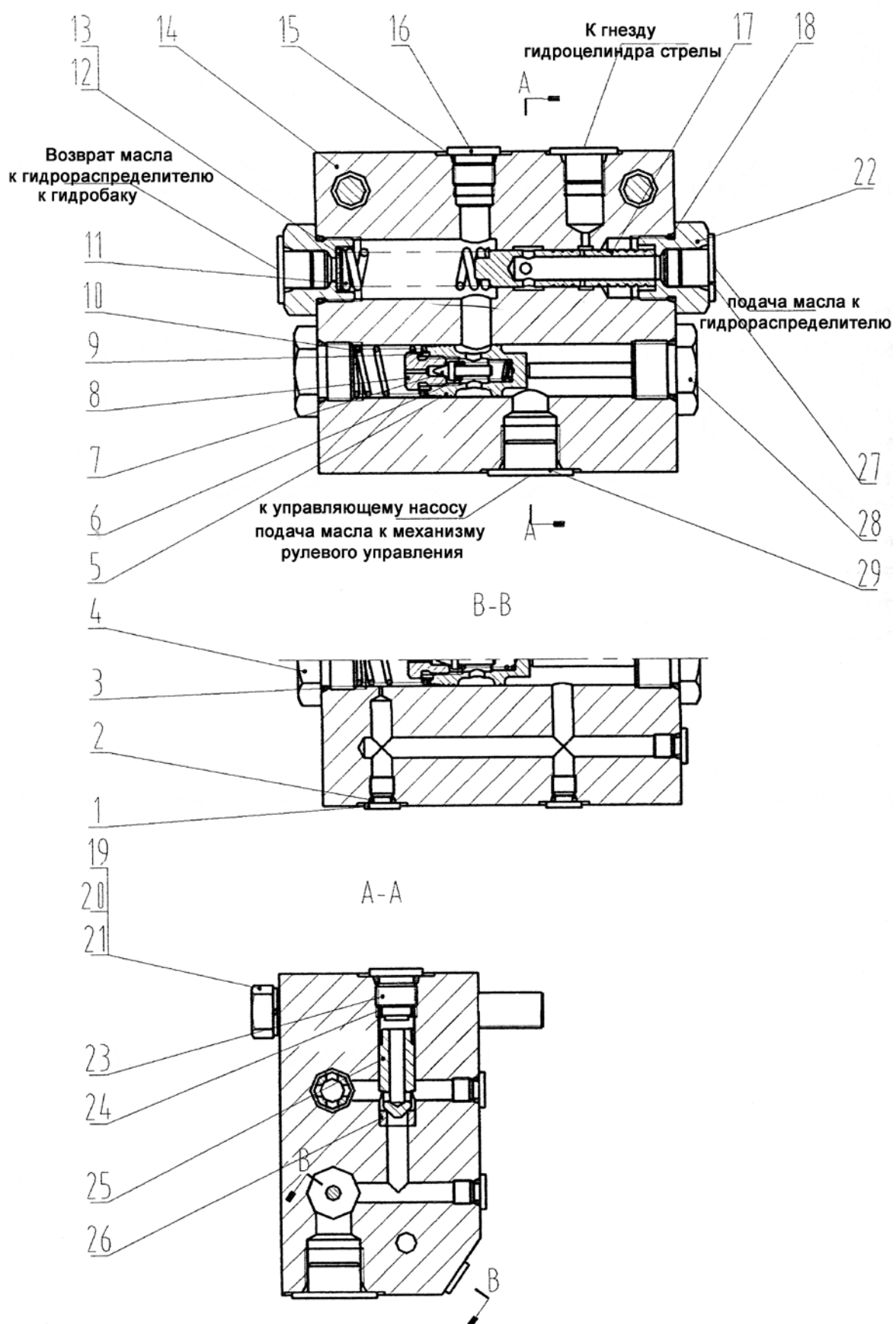
ZHF Клапан комбинированный
